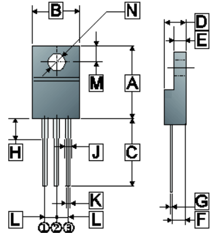
ITO-220J
