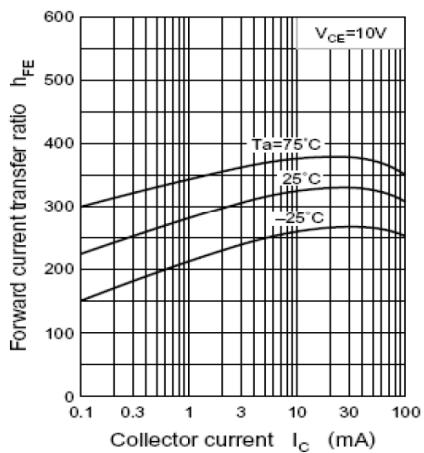
h_{FE} - I_C
