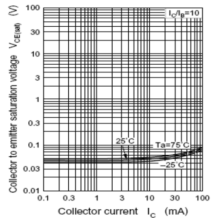
V_{CE(sat)} - I_C
