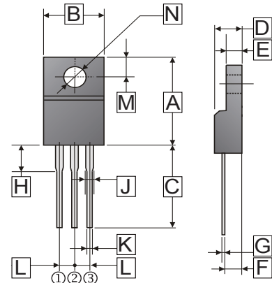
ITO-220
