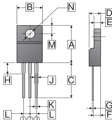
ITO-220
