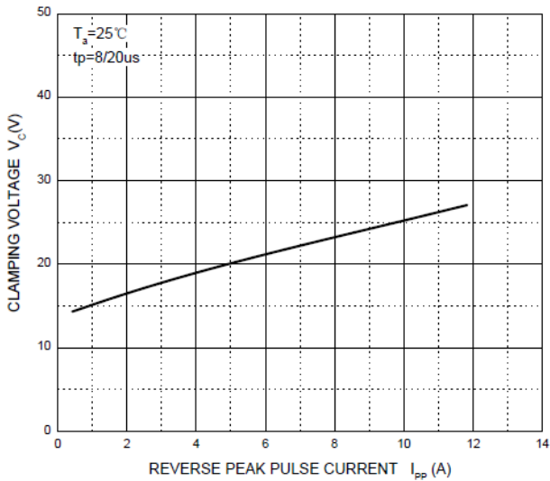
V_C — I_{PP}
