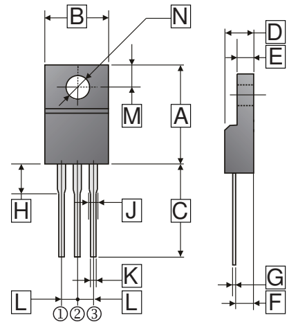
ITO-220
