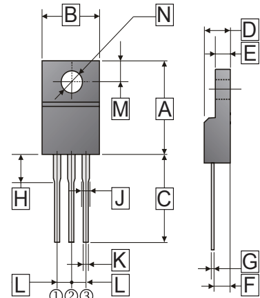
ITO-220
