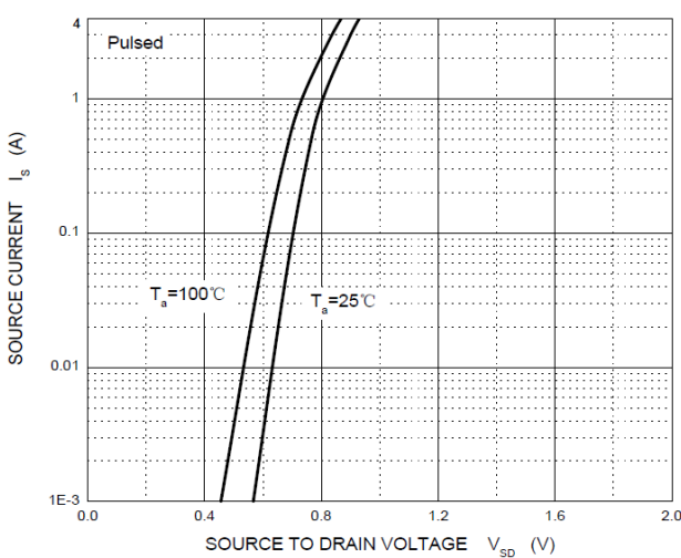
I_S — V_{SD}
