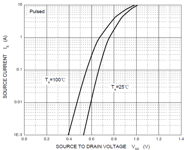
I_S — V_{SD}
