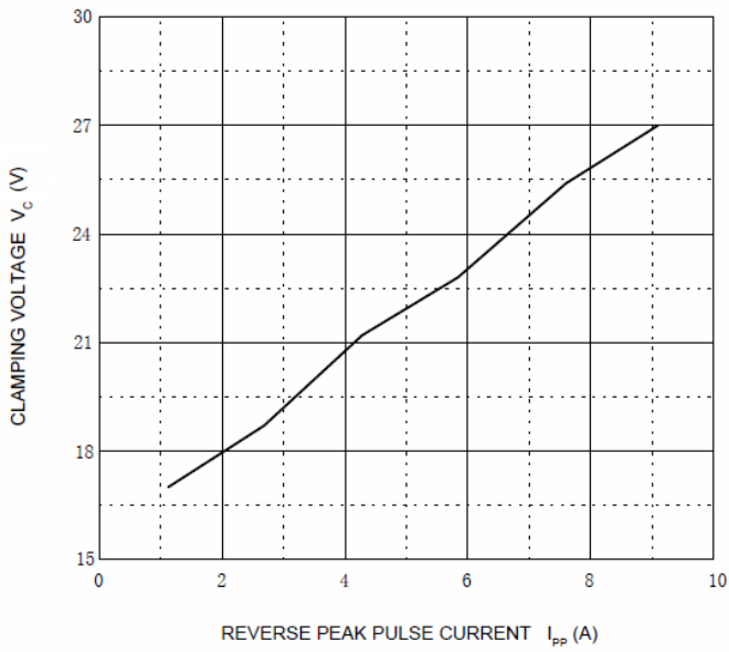
V_c — I_{pp}
