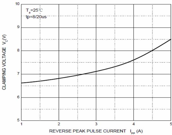
V_C — I_{PP}
