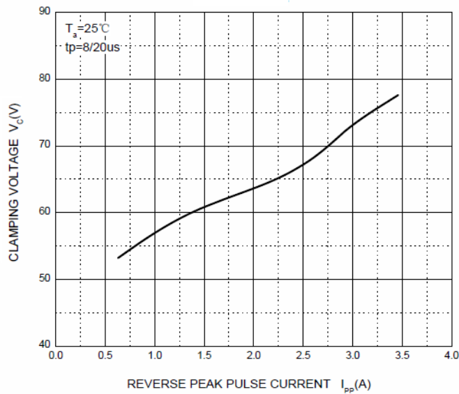
V_C — I_{PP}
